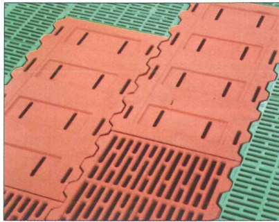
Profil 25081-400 HT, Festfläche 800x400mm
